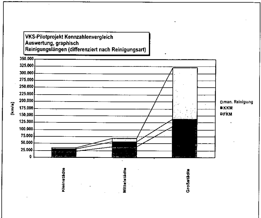
Abb. 2: Reinigungslängen
