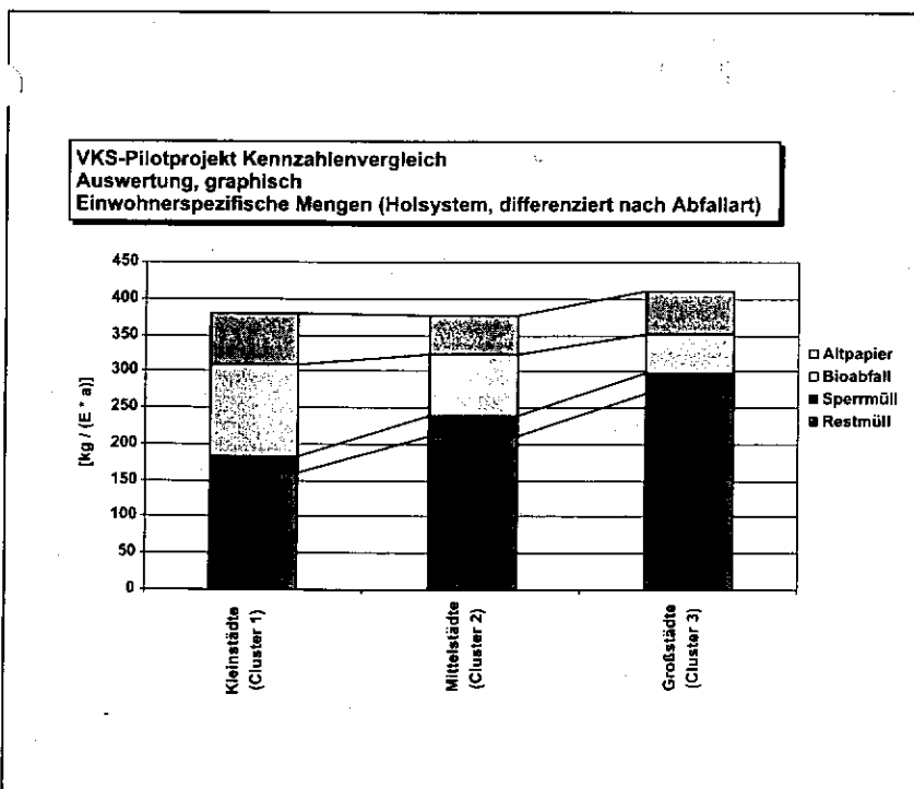
Abb. 1: Spezifische Abfallmengen
